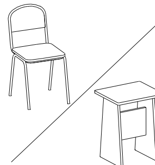
Стул на мет. каркасе ** / Табурет
